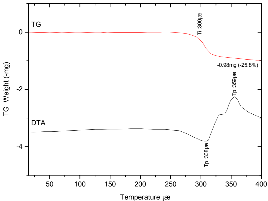
Fig. S1. TG-DTA for 1.
