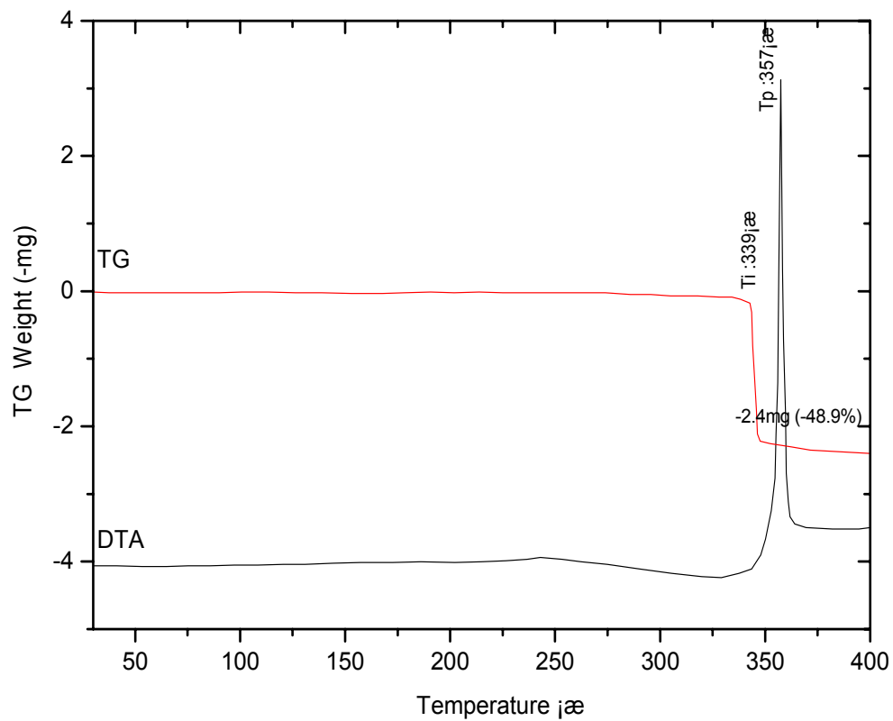
Fig. S3. TG-DTA for 3.
