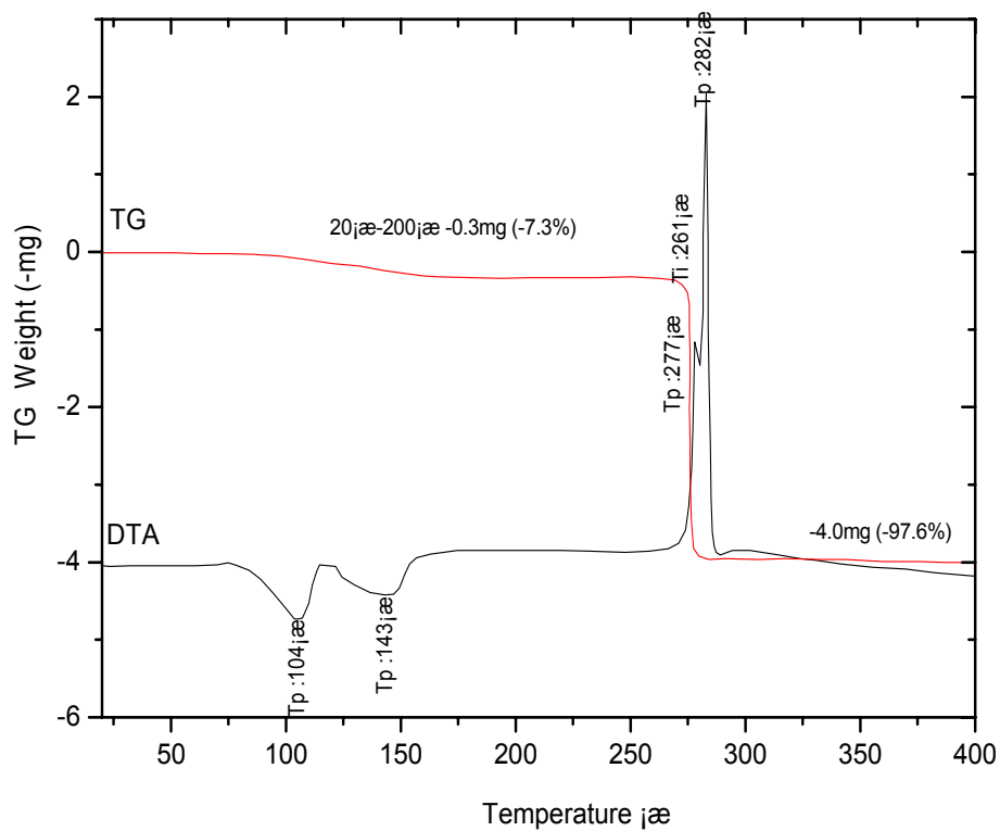
Fig. S4. TG-DTA for 4.
