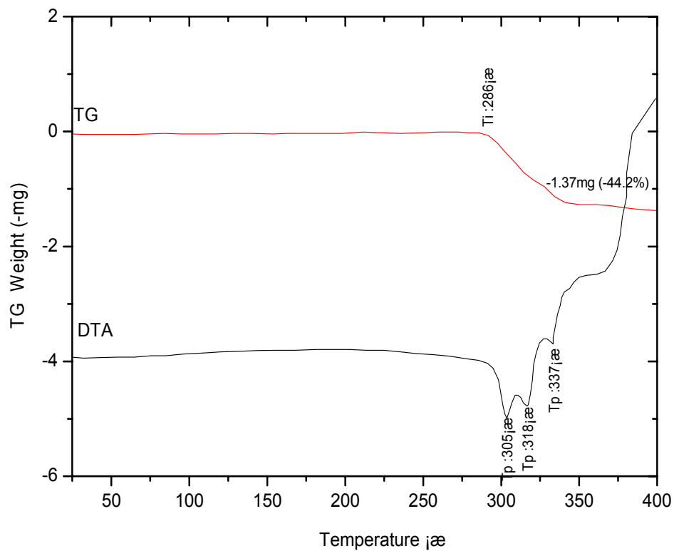
Fig. S2. TG-DTA for 2.
