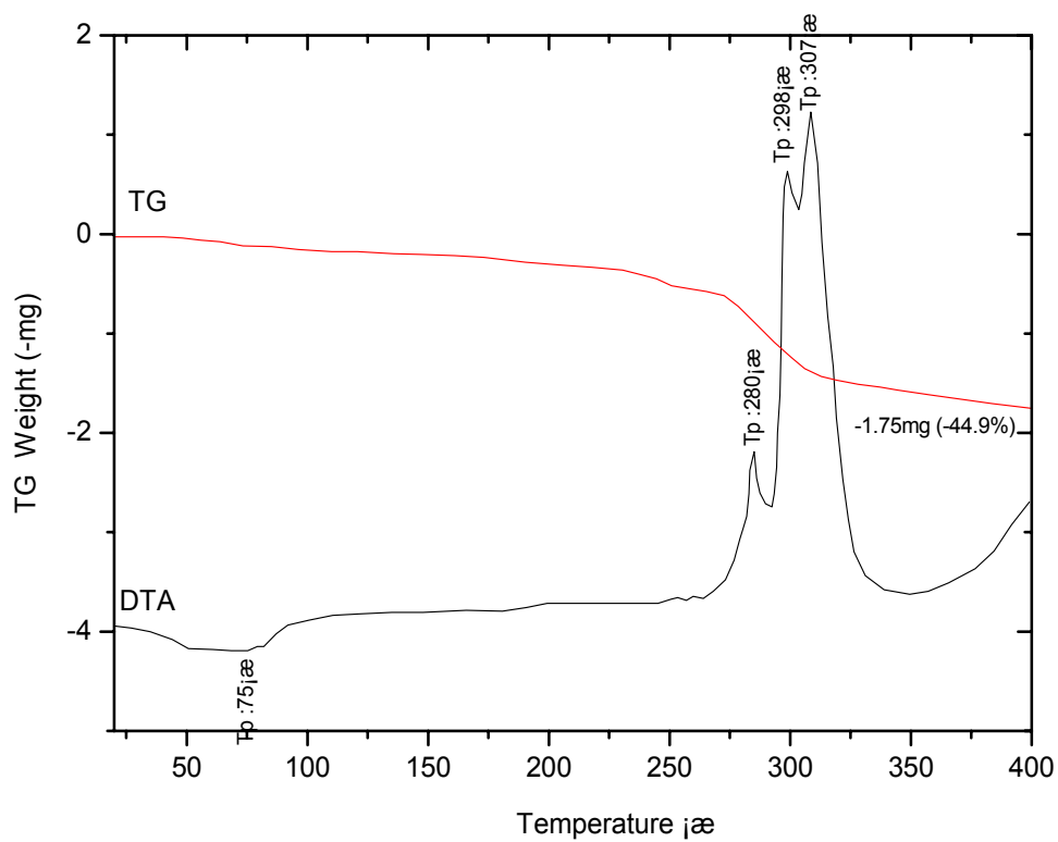
Fig. S5. TG-DTA for 5.
