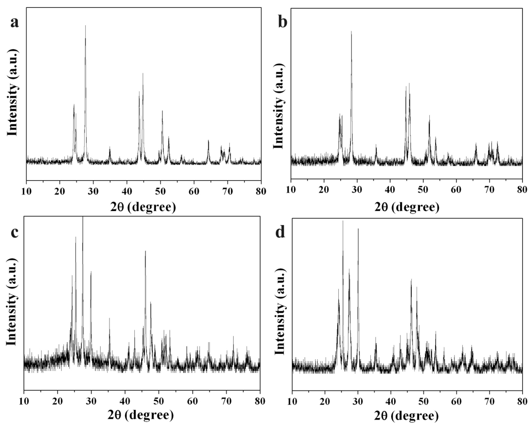
Fig. S3 XRD pattern of LnF 3 obtained at 140 °C for 20 h: (a) LaF 3 ; (b) NdF 3 ; (c) EuF 3 ; (d) GdF 3 .
