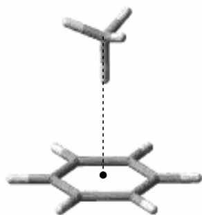
Benzene·CH 4 ( C_3 )
