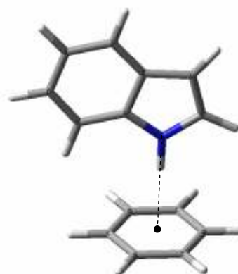
Indole·benzene T-shape ( C_1 )
