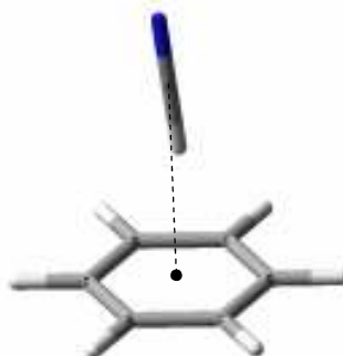
Benzene·HCN ( C_s )
