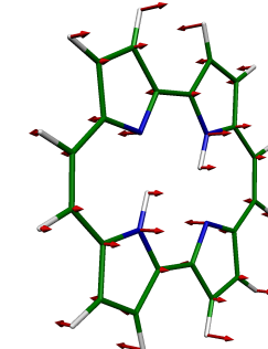
4 AU, 206 \text{cm}^{-1}
