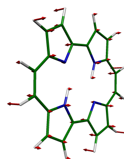
5 AU, 311 \text{cm}^{-1}
