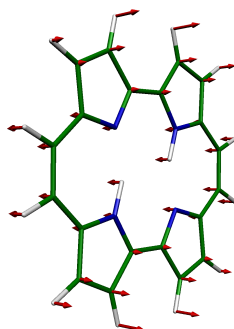
2 AU, 72 \text{cm}^{-1}
