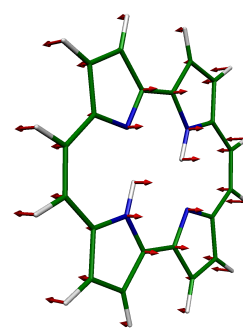
3 AU, 89 \text{cm}^{-1}
