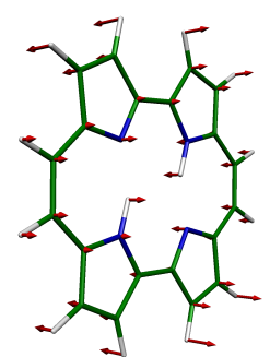
1 BG, 119 \text{cm}^{-1}
