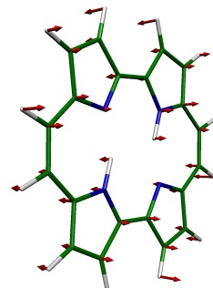
3 BG, 198 \text{cm}^{-1}
