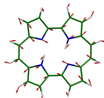
1 AG, 150 \text{cm}^{-1}
