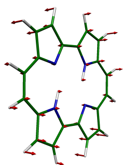
1 AU, 61 \text{cm}^{-1}
