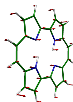
2 BG, 137 \text{cm}^{-1}
