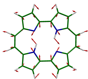
2 AG, 187 \text{cm}^{-1}
