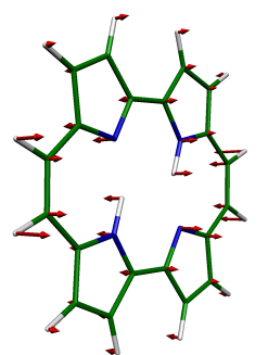
4 BG, 209 \text{cm}^{-1}
