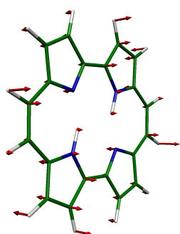
6 AU, 320 \text{cm}^{-1}
