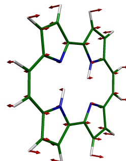
5 BG, 399 \text{cm}^{-1}
