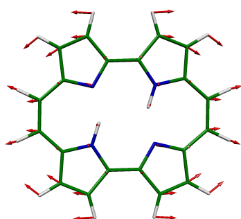
4 AG, 370 \text{cm}^{-1}
