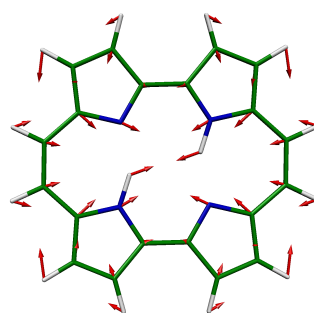
3 AG, 347 \text{cm}^{-1}
