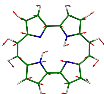
3 BU, 391 \text{cm}^{-1}
