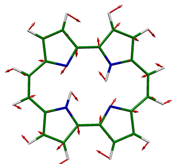
5 AG, 491 \text{cm}^{-1}
