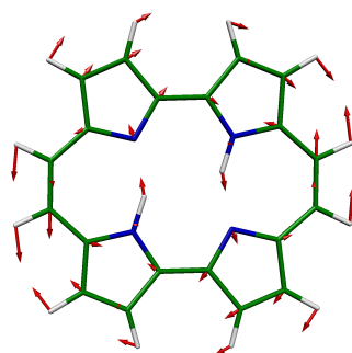
6 AG, 610 \text{cm}^{-1}
