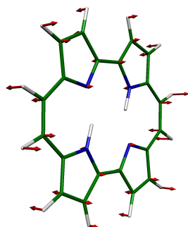
7 AU, 512 \text{cm}^{-1}
