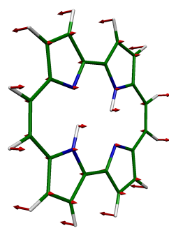
12 AU, 765 \text{cm}^{-1}
