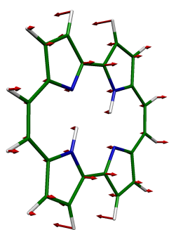
8 AU, 640 \text{cm}^{-1}
