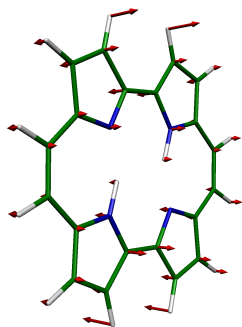
7 BG, 644 \text{cm}^{-1}
