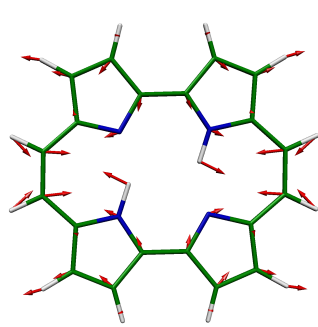
7 AG, 674 \text{cm}^{-1}
