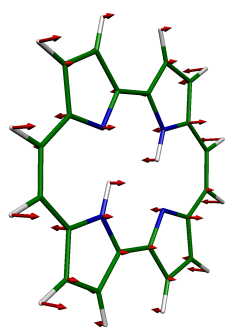
8 BG, 673 \text{cm}^{-1}
