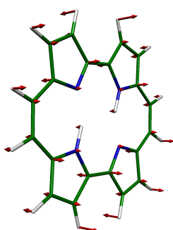
11 AU, 726 \text{cm}^{-1}
