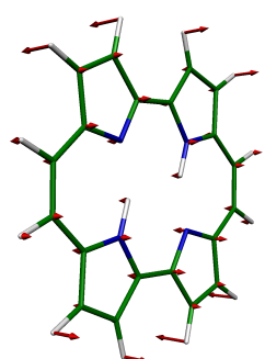
10 AU, 714 \text{cm}^{-1}
