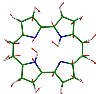
6 BU, 673 \text{cm}^{-1}
