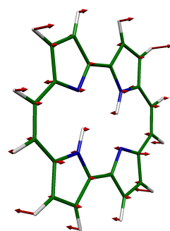
10 BG, 718 \text{cm}^{-1}
