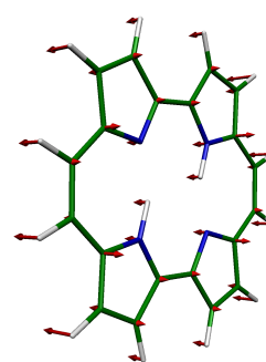
9 AU, 674 \text{cm}^{-1}
