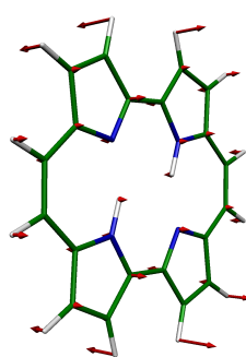
9 BG, 713 \text{cm}^{-1}
