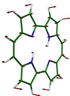
13 AU, 796 \text{cm}^{-1}
