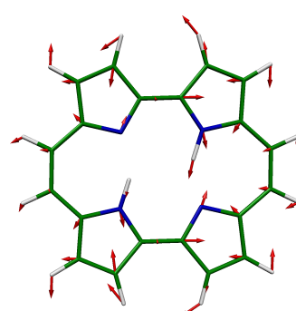
8 BU, 896 \text{cm}^{-1}
