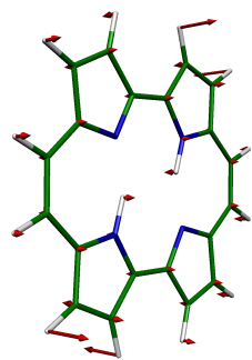
15 BG, 904 \text{cm}^{-1}
