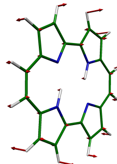
16 AU, 905 \text{cm}^{-1}
