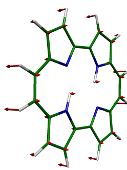
14 AU, 834 \text{cm}^{-1}
