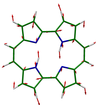
9 AG, 877 \text{cm}^{-1}
