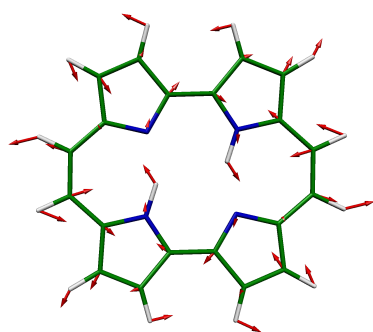
8 AG, 833 \text{cm}^{-1}
