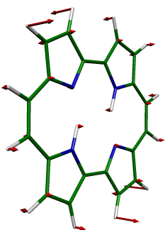
14 BG, 897 \text{cm}^{-1}
