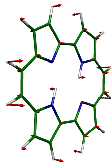
13 BG, 832 \text{cm}^{-1}
