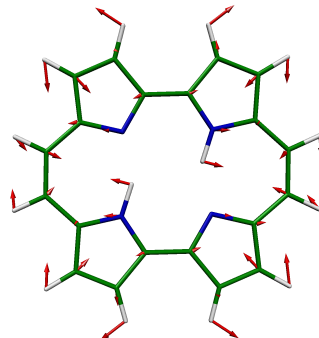
10 AG, 989 \text{cm}^{-1}
