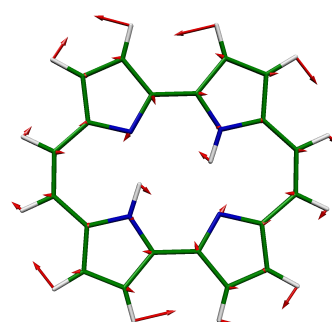
13 AG, 1083 \text{cm}^{-1}
