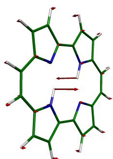
16 BG, 933 \text{cm}^{-1}
