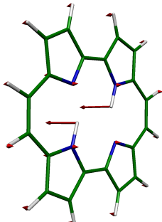
18 AU, 999 \text{cm}^{-1}
