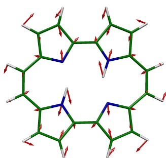
11 AG, 994 \text{cm}^{-1}
