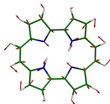
12 AG, 1016 \text{cm}^{-1}
