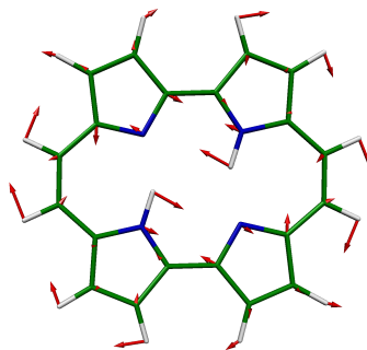
18 AG, 1292 \text{cm}^{-1}
