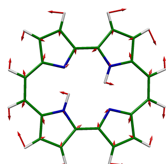
16 AG, 1193 \text{cm}^{-1}
