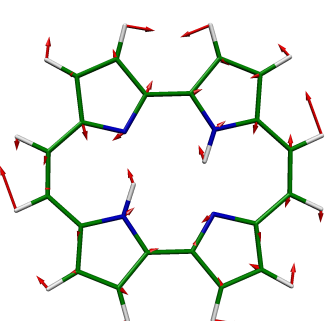
15 BU, 1210 \text{cm}^{-1}
