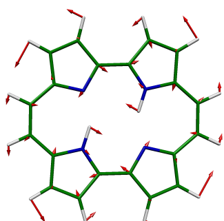
15 AG, 1142 \text{cm}^{-1}
