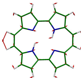
17 AG, 1240 \text{cm}^{-1}
