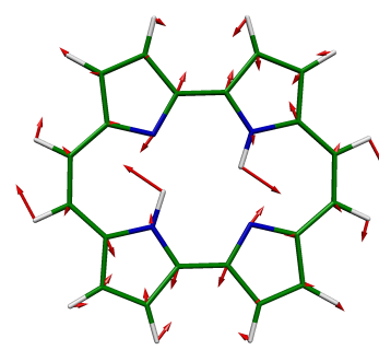
19 AG, 1312 \text{cm}^{-1}
