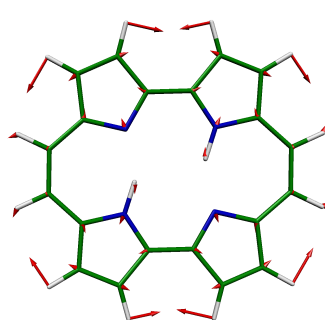
14 AG, 1092 \text{cm}^{-1}
