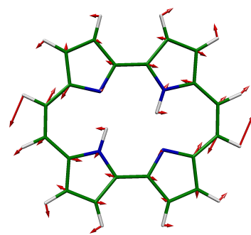
28 AG, 1592 \text{cm}^{-1}
