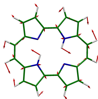
26 AG, 1532 \text{cm}^{-1}
