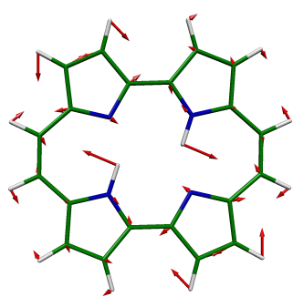
27 AG, 1563 \text{cm}^{-1}
