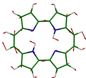
29 AG, 1613 \text{cm}^{-1}
