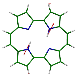
31 AG, 2895 \text{cm}^{-1}
