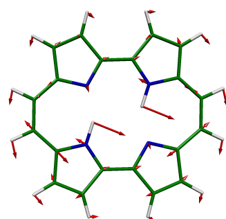
29 BU, 1631 \text{cm}^{-1}
