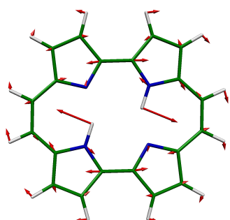
30 AG, 1663 \text{cm}^{-1}
