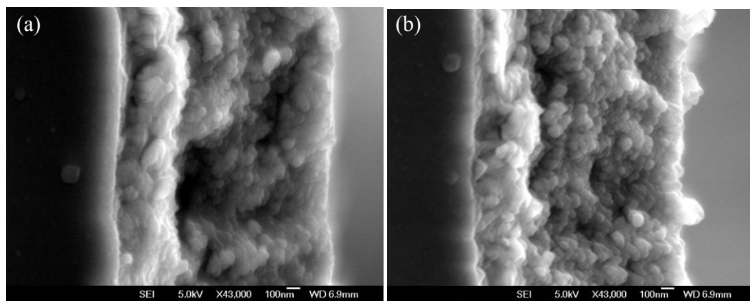
Fig. S1 FEG-SEM cross-sectional images of a configuration TiO 2 /P3HT (a) and TiO 2 /TAA/P3HT (b).
