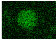
Fe K
