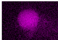
F K
