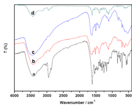
Fig. S2 FT-IR spectra of (a) 3a; (b) 3b; (c) 3c; (d) the neat chiral salen Mn(III) complex 2
