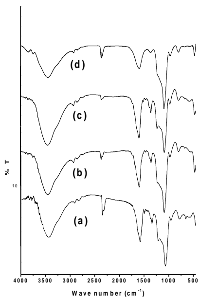
Fig. E FT-IR spectra of (a) SiMCM-48, (b) CeMCM-48(Si/Ce 40), (c) VMCM-48(Si/V 40), (d) ZrMCM-48(Si/Zr 40)
