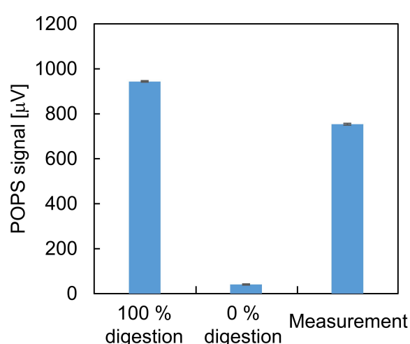
(d) 77 kPa
