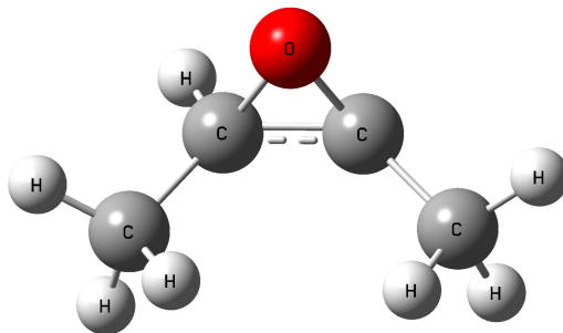
Cis-2,3-epoxybutane-H 1
