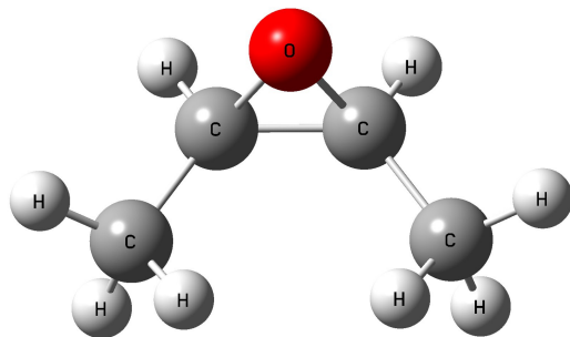
Cis-2,3-epoxybutane
