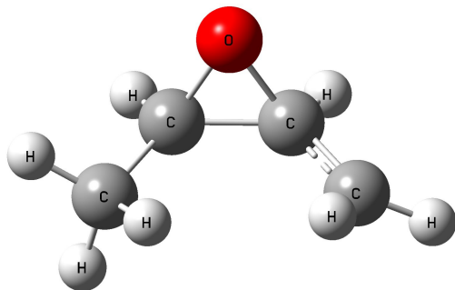
Cis-2,3-epoxybutane-H 2
