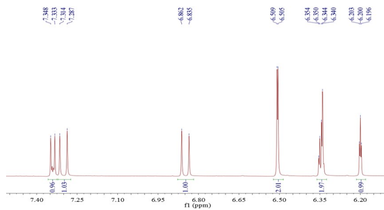
A. 1 H-NMR
