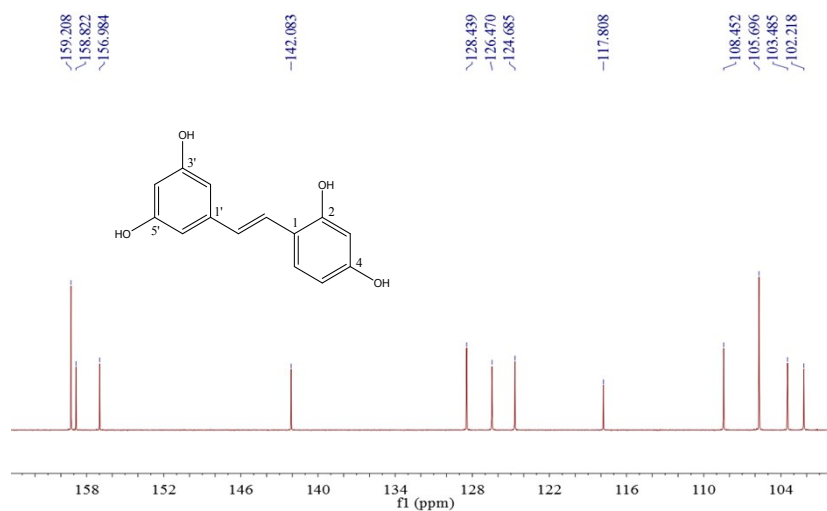
B. 13 C-NMR
