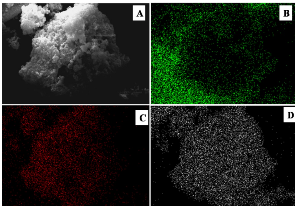
Fig. S5 Elemental mapping of ZSs@1rGO.
