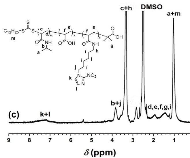
Fig. S2 ^1\text{H} NMR spectra of (a) DDMAT, (b) P(NIPAM- co -AA) and (b) P(NIPAM- co -AA- co -NIA).
