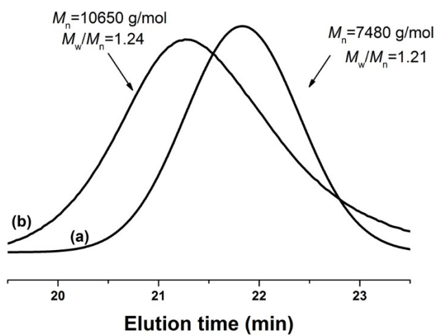
Fig. S3 GPC traces of (a) P(NIPAM- co -AA) and (b) P(NIPAM- co -AA- co -NIA).
