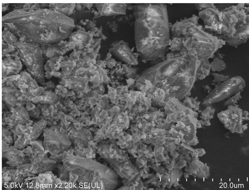
Fig. S2 SEM images of Co/Ni-MOF-74
