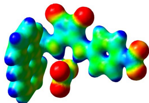
4-NO 3 -
