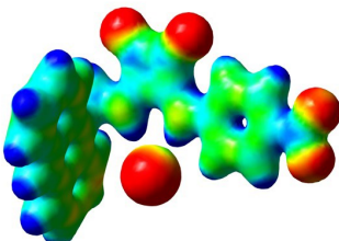
4-Br -
