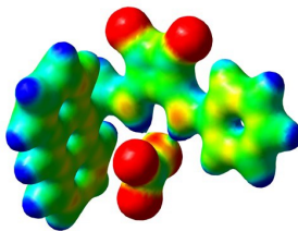
1-NO 3 -
