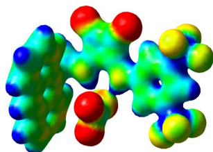
2-NO 3 -
