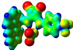
2-NO 3 -
