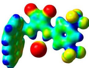
3-Br -
