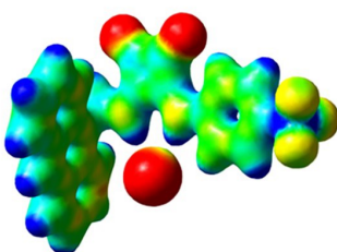
2-Br -
