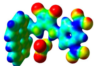
5-NO 3 -
