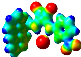
8-Cl -
