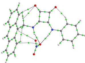
1-NO 3 -
