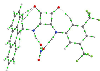
3-NO 3 -
