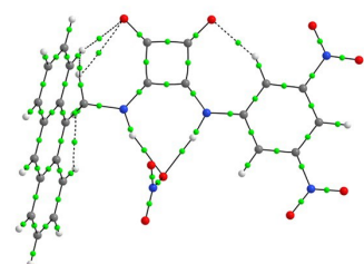
5-NO 3 -
