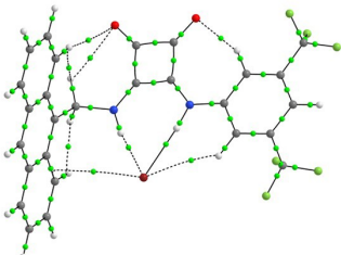
3-Br
