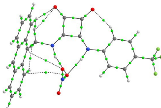
2-NO 3 -
