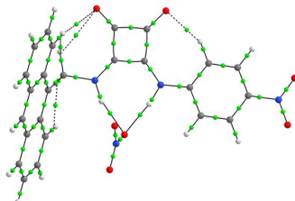
4-NO 3 -
