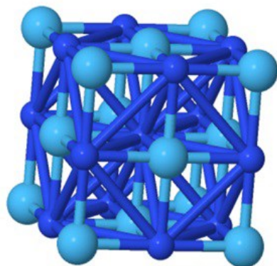
\delta -Hf(III)N
