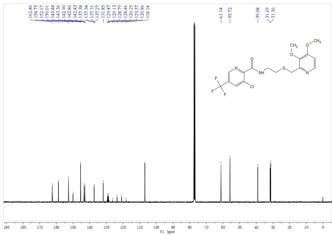
Fig. S29 13 C NMR spectra of compound E10
