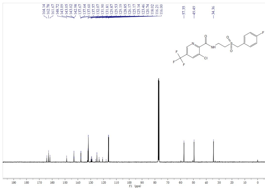
Fig. S80 13 C NMR spectra of compound F1
