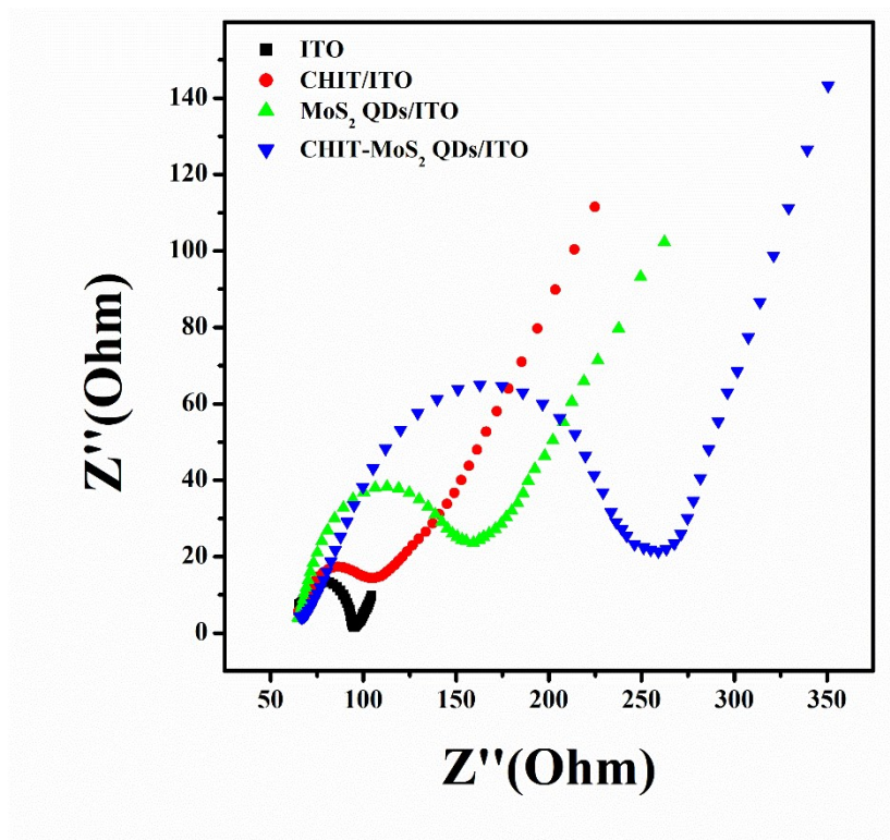
Figure S1. EIS of ITO, CHIT/ITO, MoS 2 QDs/ITO and CHIT-MoS 2 QDs /ITO.
