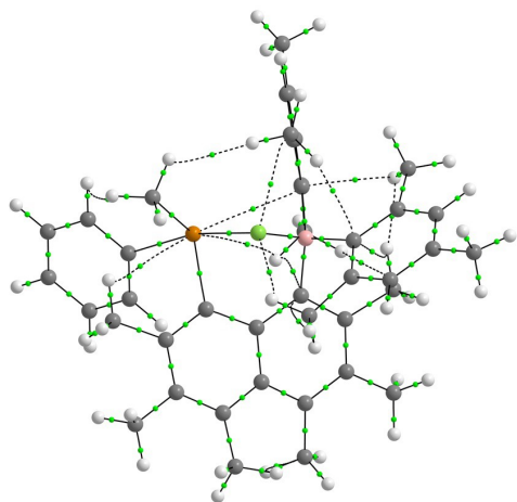
4\text{CH}_3\cdots\text{F}^-
