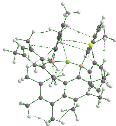
5\text{H},\text{CH}_3\cdots\text{F}^-
