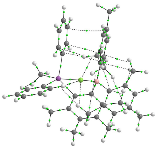
6\text{CH}_3\cdots\text{F}^-
