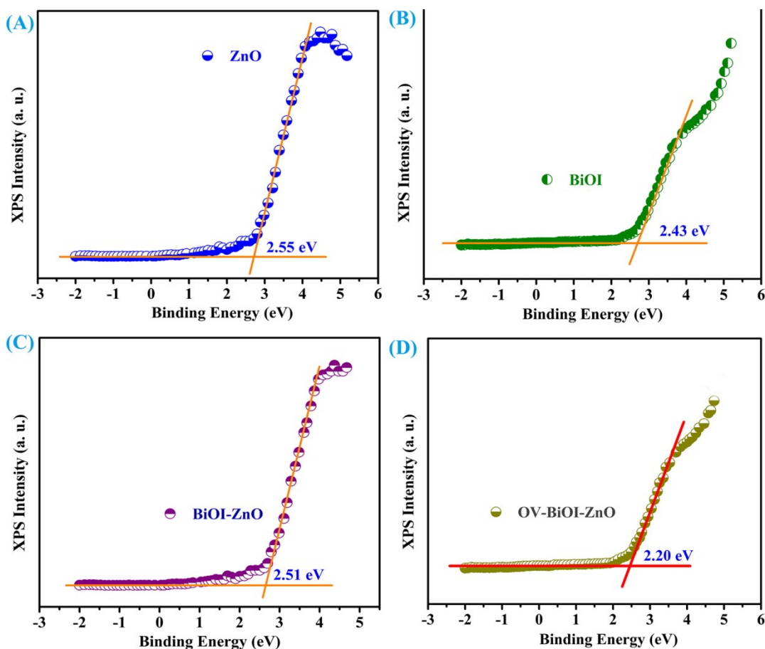
Fig. S1 The VB spectra of ZnO (A), BiOI (B), BiOI-ZnO (C) and OV-BiOI-ZnO (D) heterostructures.
