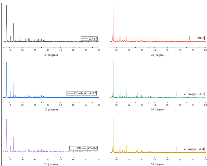
Fig. S2 XRD patterns of ZIF-67@ZIF-8, ZIF-67 and ZIF-8
