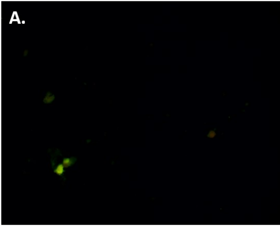
ZnO
