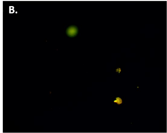
ZnSe
