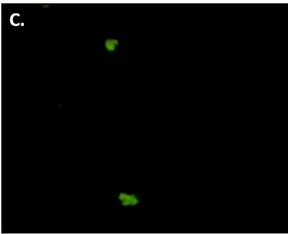
ZnS:Mn
