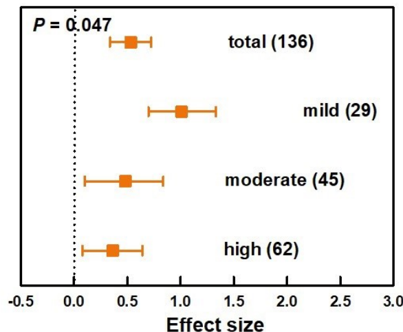
(d) Vegetation type
