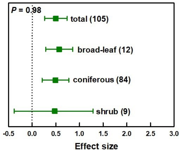
(d) Vegetation type
