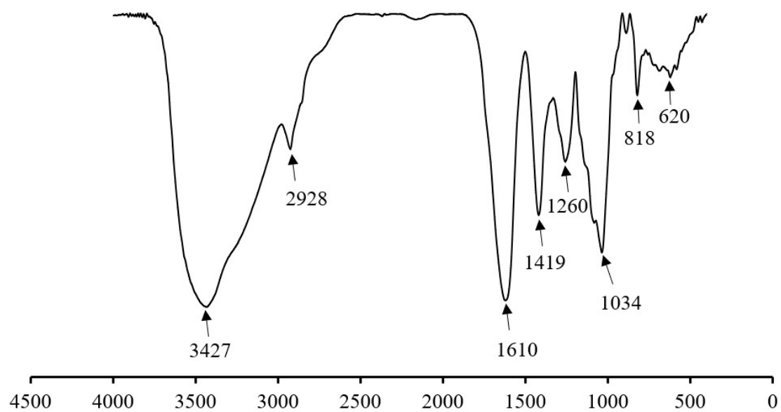
Fig. S1 The IR spectra of UPP
