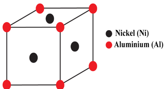
Fig. S1. Ni 3 Al (L 12 ) crystal structure
