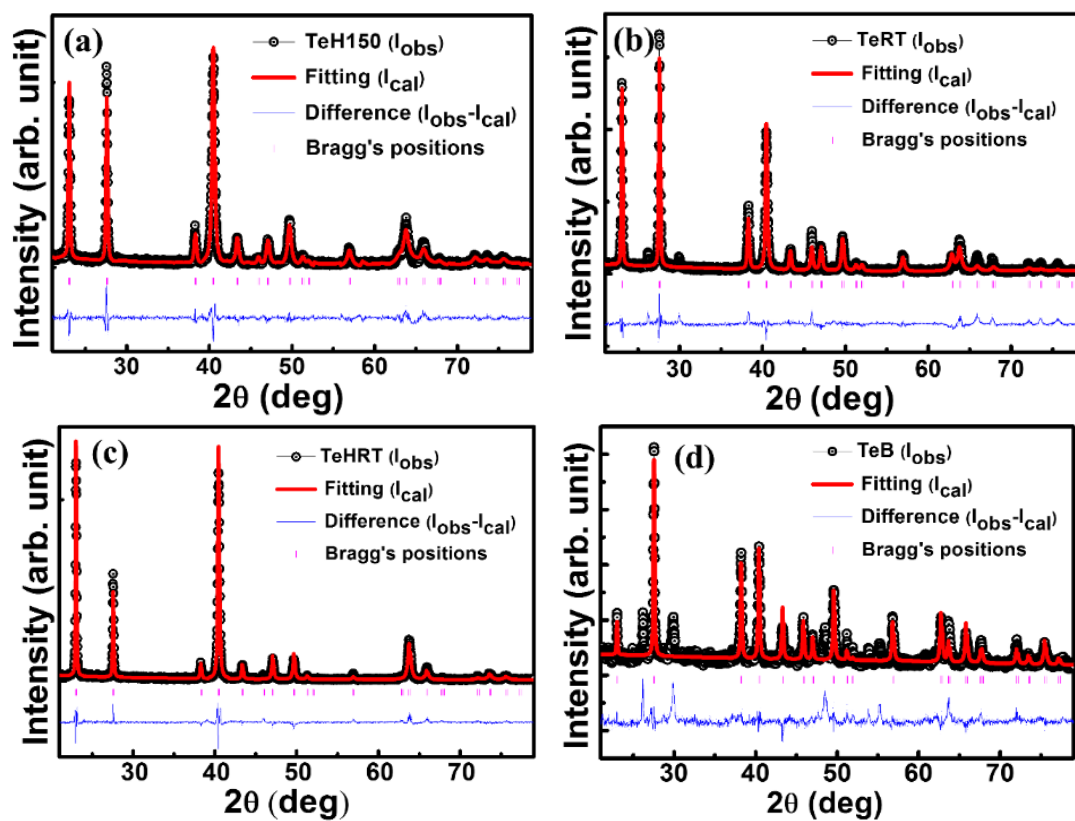
Fig. S1 Rietveld refinement of (a) TeH150, (b) TeRT, (c) TeHRT and (d) TeB.
