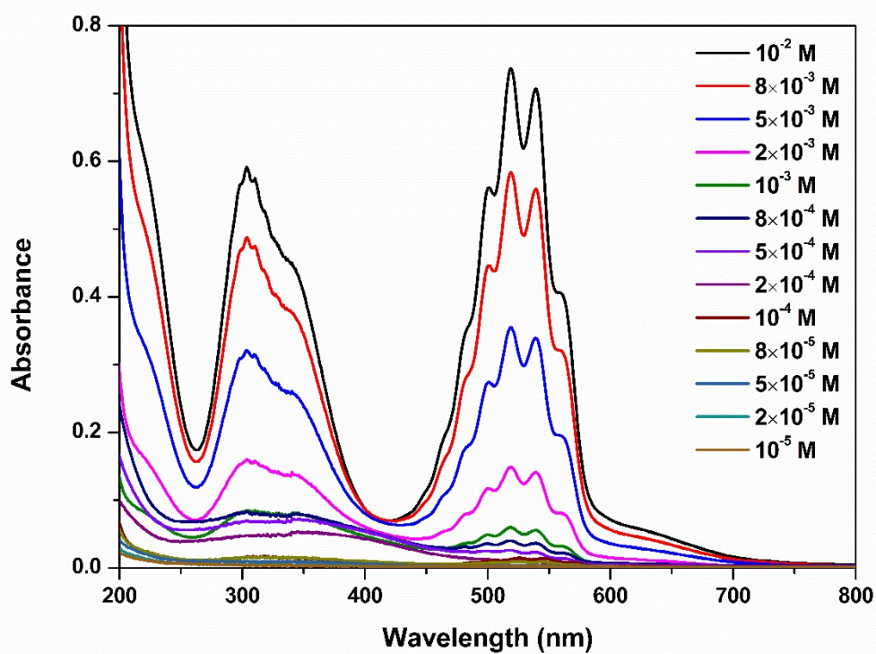
Fig S2: Absorption spectra of \text{KMnO}_4 ( 10^{-2} - 10^{-5} M)
