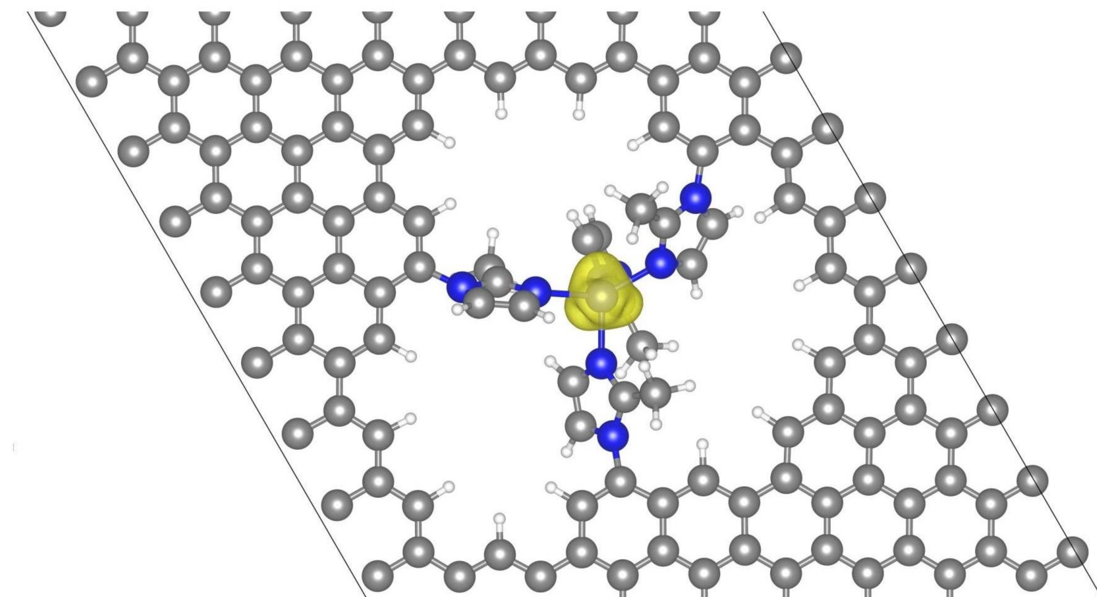
(d) Fe-(mIM) 4
