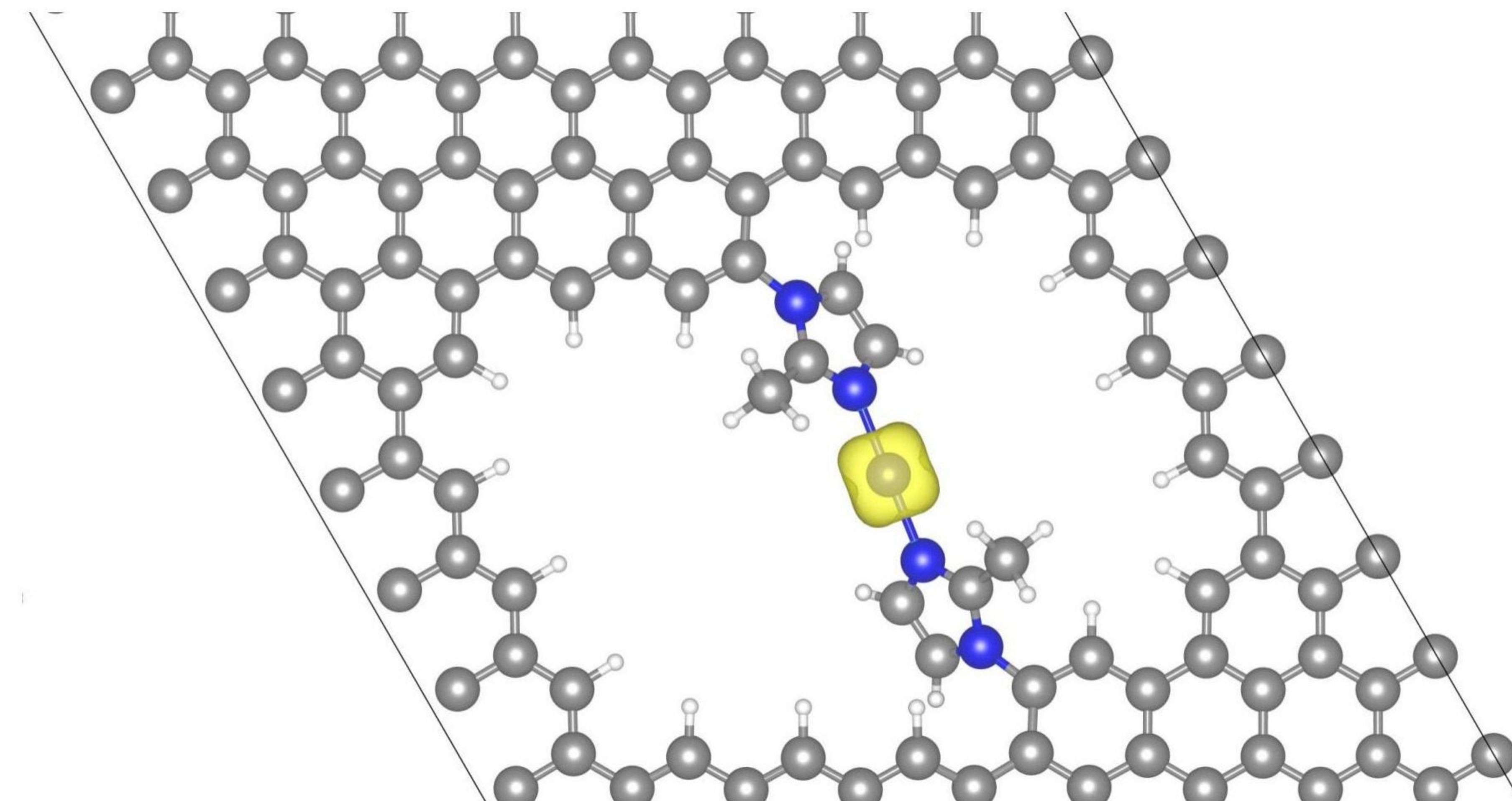
(d) Fe-(mIM) 4
