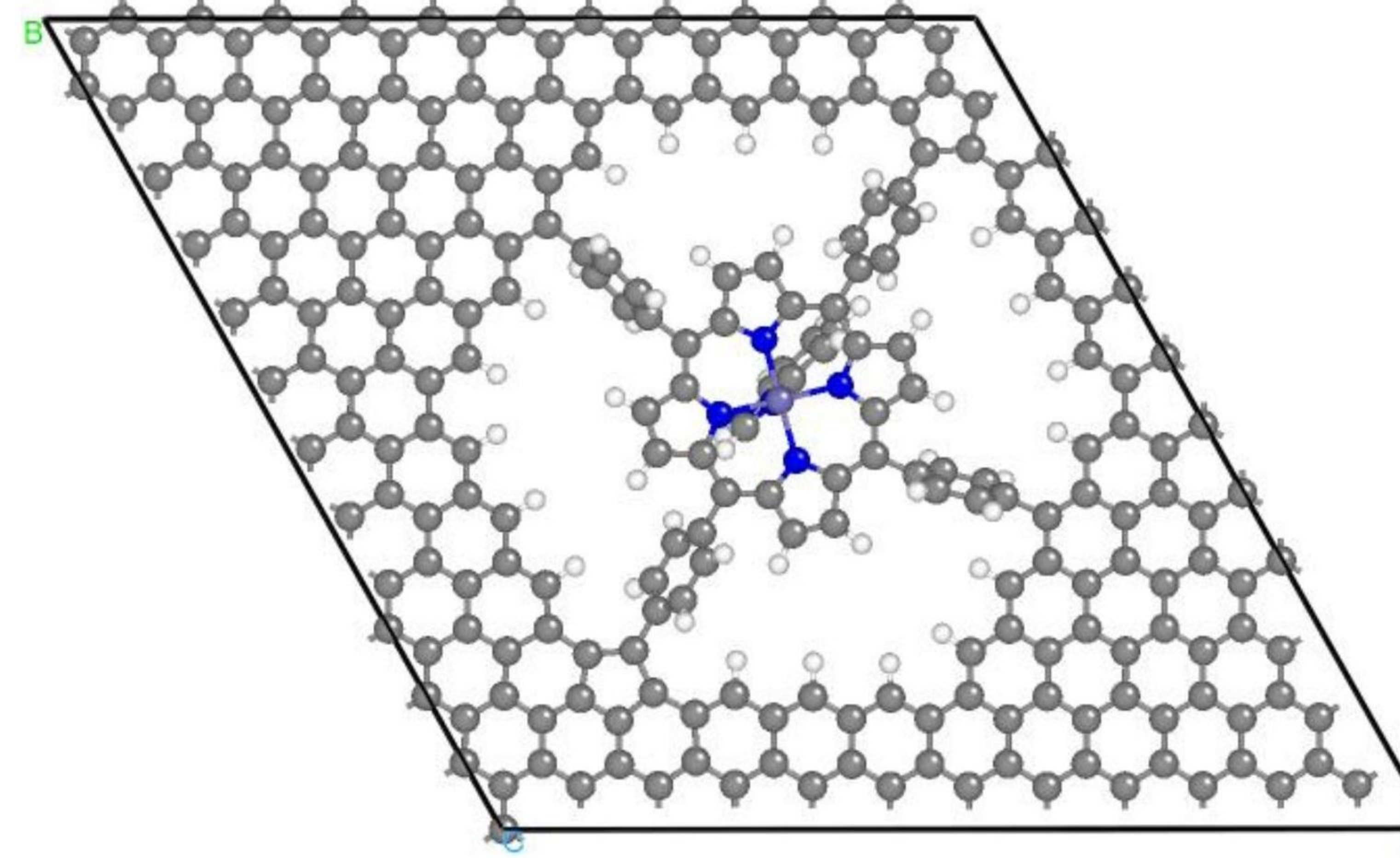
(d) Fe-TCPP_bIm_N
