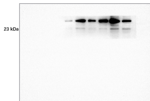
Fig 6B C-Caspase-1
