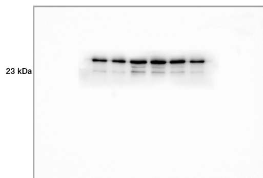
Fig 5D C-Caspase-1
