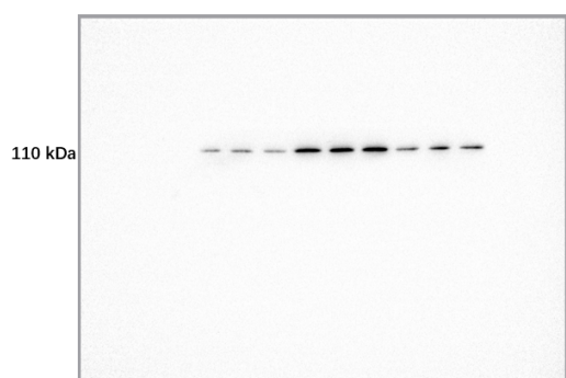
Fig 4B NLRP3
