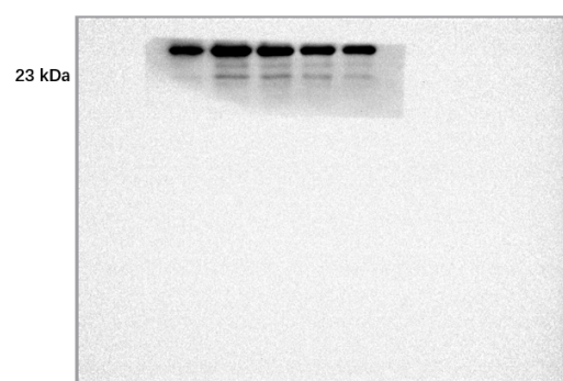
Fig 5K C-Caspase-1
