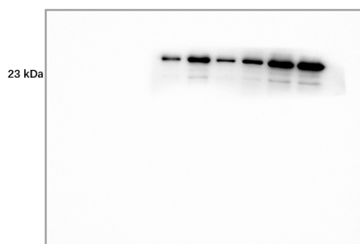
Fig 6G C-Caspase-1
