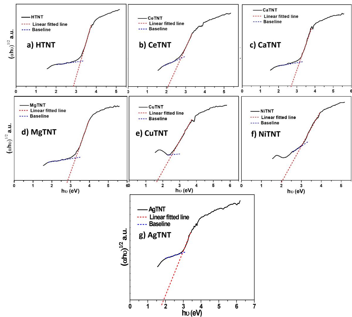
Fig S2: The tauc plots for a) HTNT, b) CeTNT, c) CaTNT, d) MgTNT, e) CuTNT, f) NiTNT and g) AgTNT
