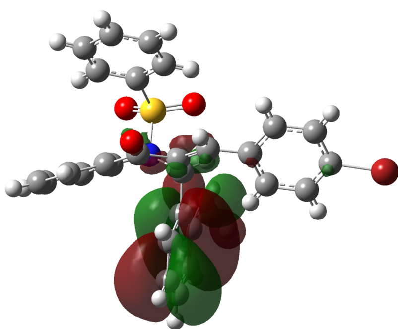
HOMO (-178.62 kcal/mol)
