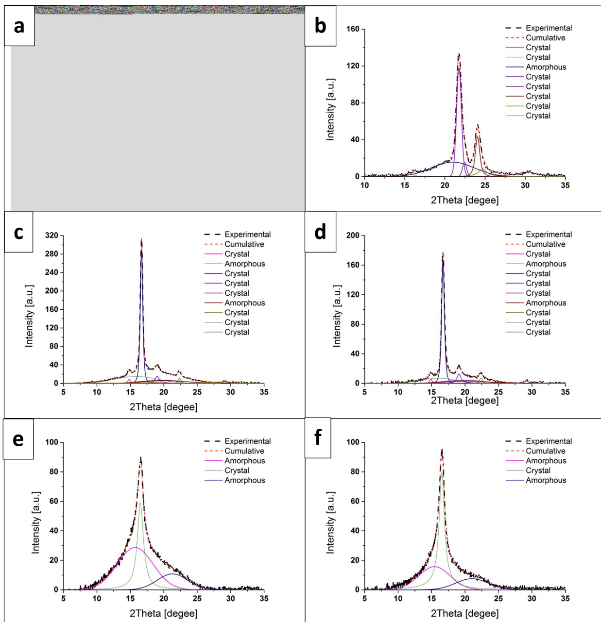
Figure S3. WAXS scattering profiles of: a) PCL_10%_24h, b) PCL_30%_24h, c) PLCL_2%_5 min, d) PLCL_10%_10 min, e) PLLA_2%_5 min, f) PLLA_6%_10 min with fitting.
