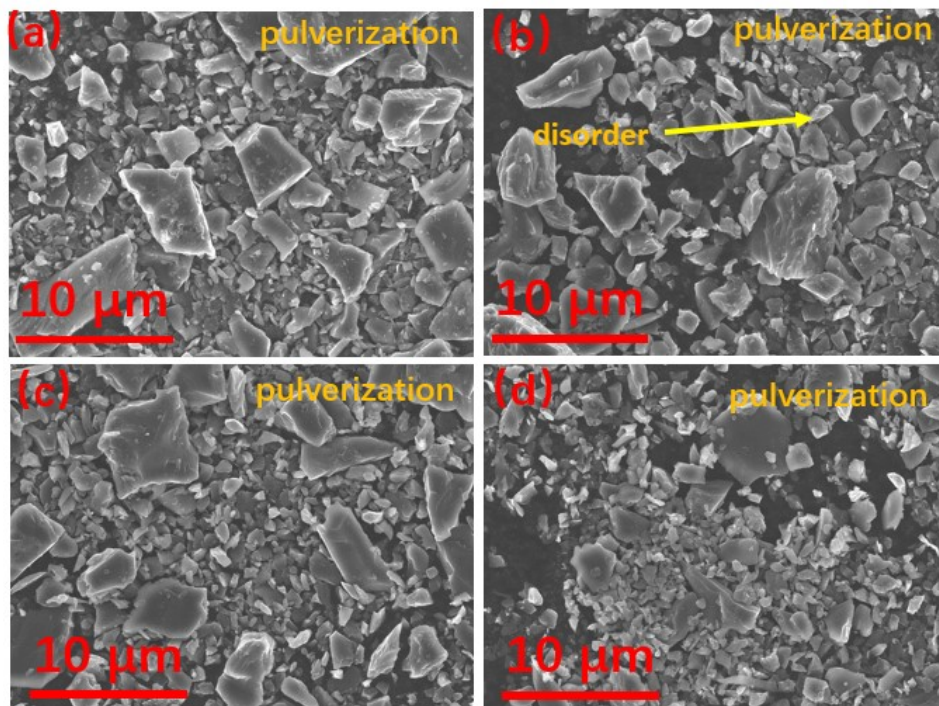
Fig.S2 SEM images about WYM-800 (a), WYM-1000 (b), WYM-1200 (c), WYM-1400 (d)
