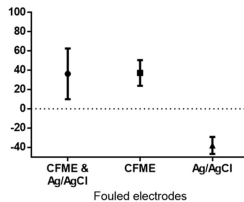
(d) \Delta E_{p,post} - \Delta E_{p,pre} (mV)
