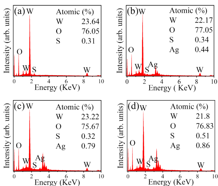
Fig. S1 SEM-EDS spectra: (a) S-WO 3 , (b) SWAS50, (c) SWAS100, and (d) SWAS150.
