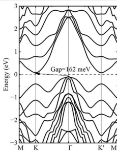
(b) CrSiGeP 4
