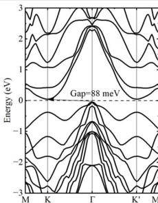
(c) CrSiGeAs 4
