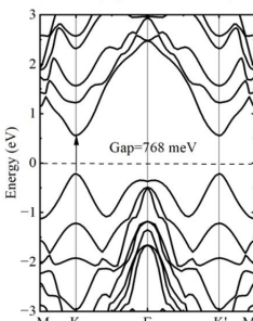
(e) WSiGeP 4
