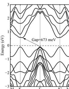
(f) WSiGeAs 4
