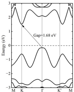
(d) WSiGeN 4
