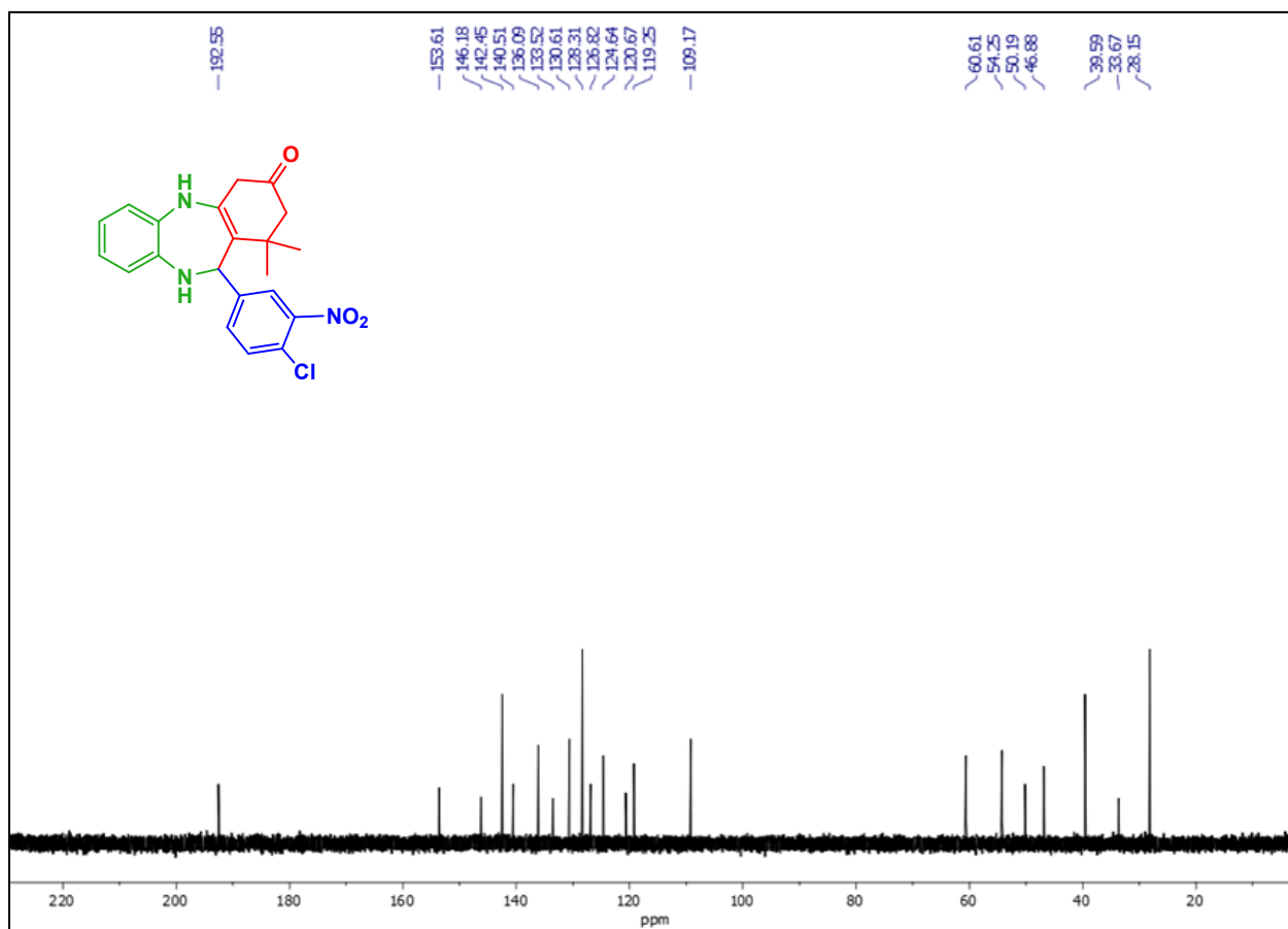
^{13}\text{C} -NMR spectra of 4e
