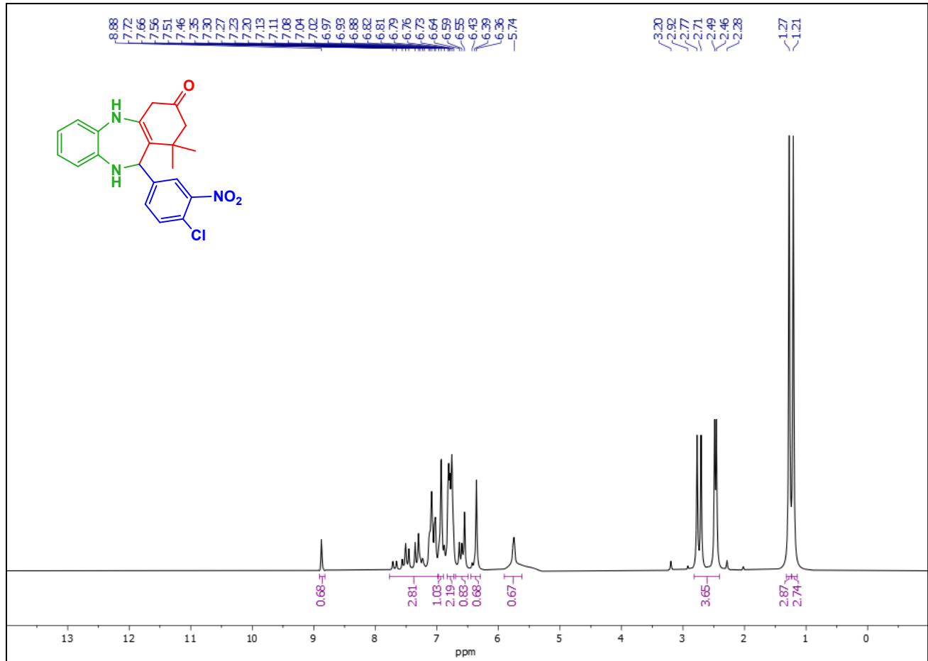
1 H-NMR spectra of 4e
