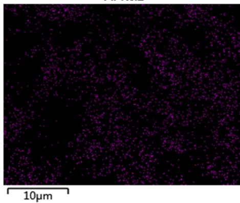
Al Kα1
