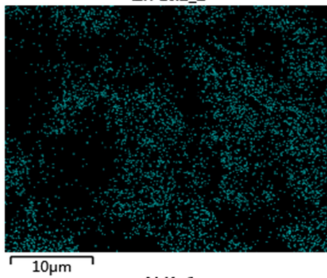
Al Kα1
