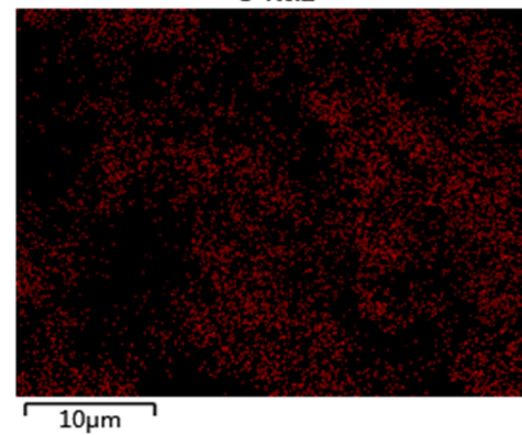
O Kα1
