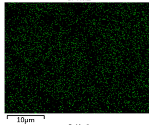
O Kα1
