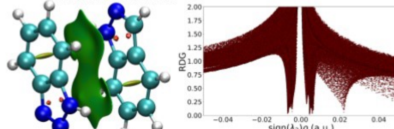
Indazole-Benzotriazole
