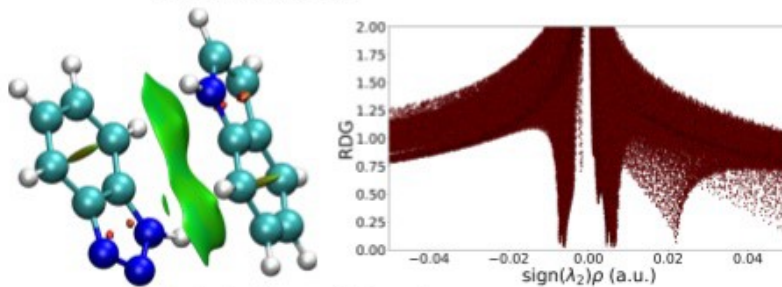
Indole-Benzotriazole
