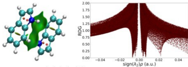
Indole-Indole
