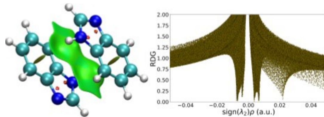
Benzimidazole-Benzimidazole
